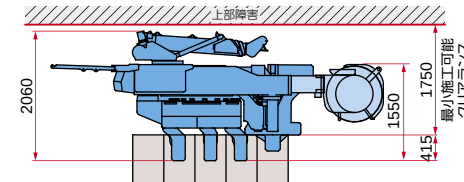
500mm施工時
