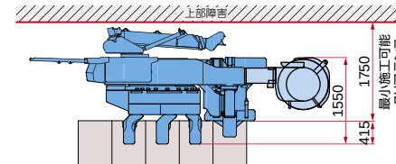
600mm施工時
